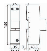
Rozměry DBM 1 440
