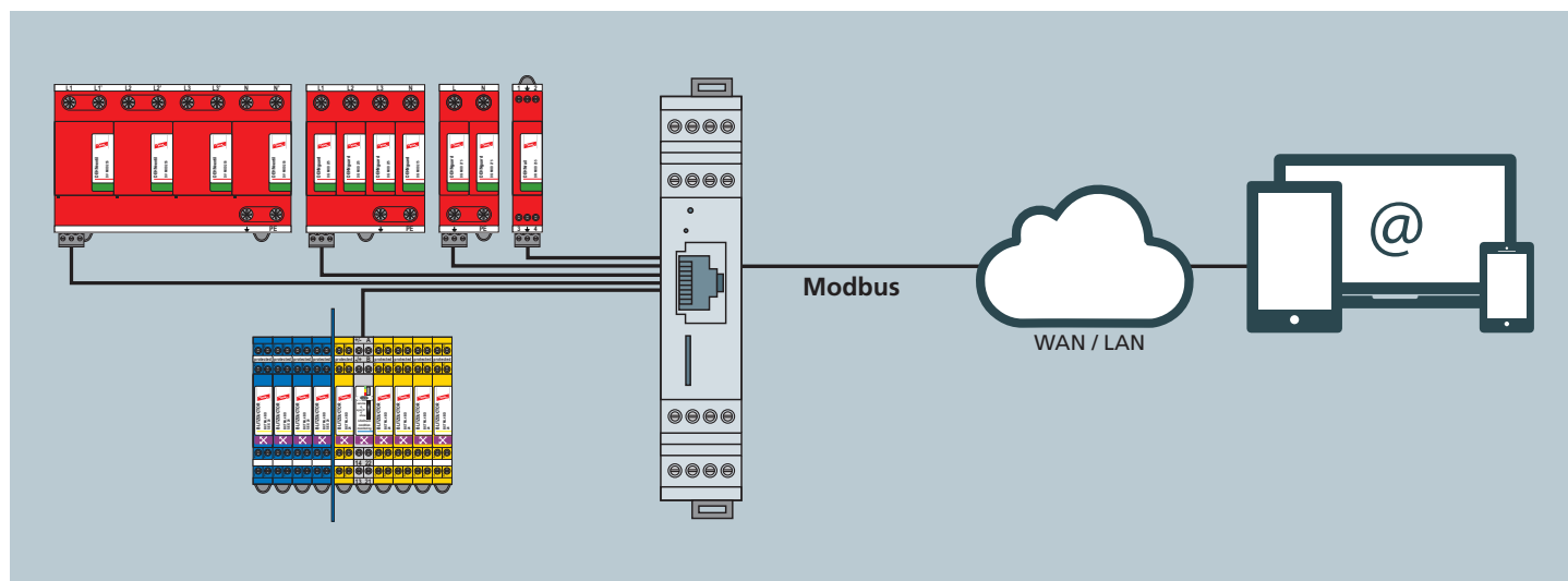
Složení celkového systému DEHNrecord Alert se svodiči přepětí řady Red/Line® a Yellow/Line®
