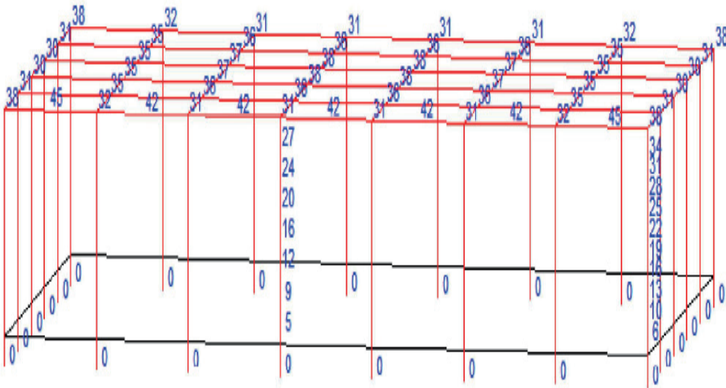
Obr. 3a Datové centrum – výpočet dostatečné vzdálenosti pro holý drát
