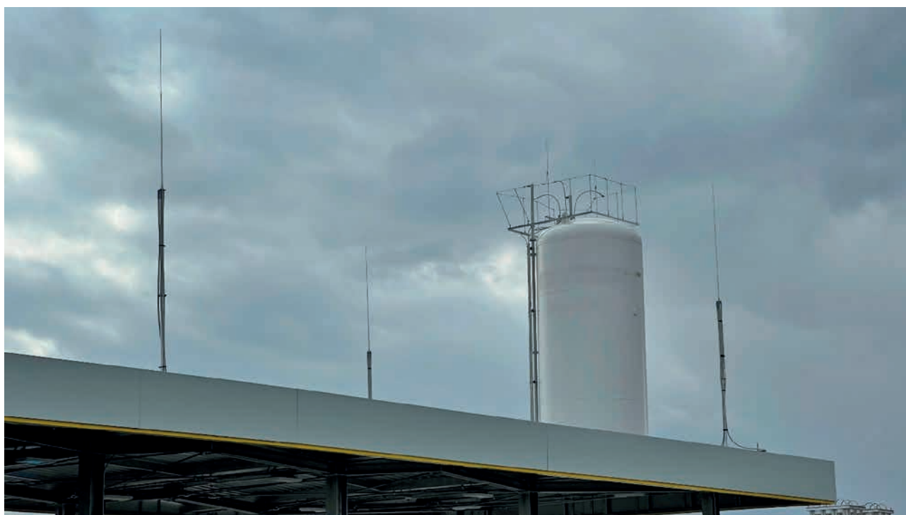
Obrázek 3 – Detail jímací soustavy
